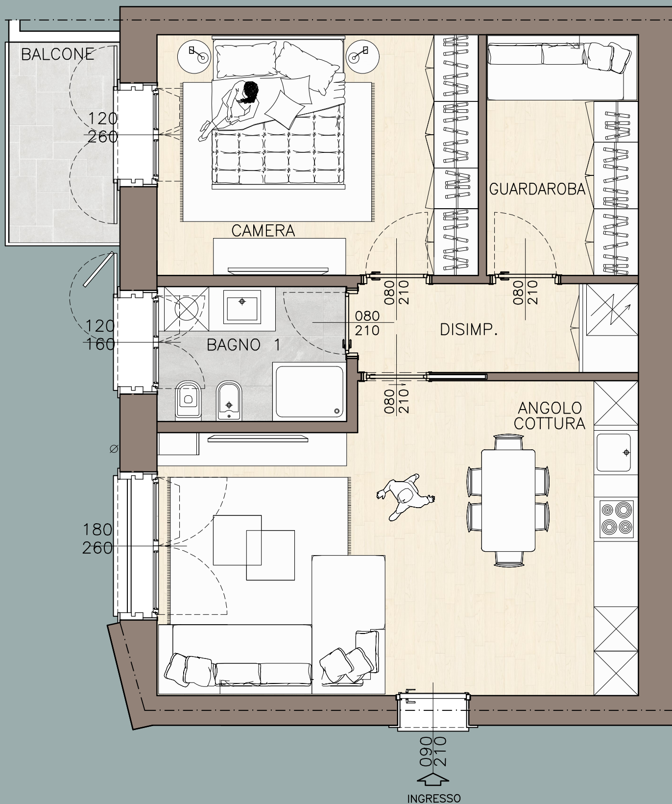
Pianta Appartamento B6 - opzione 2 scala 1:50
