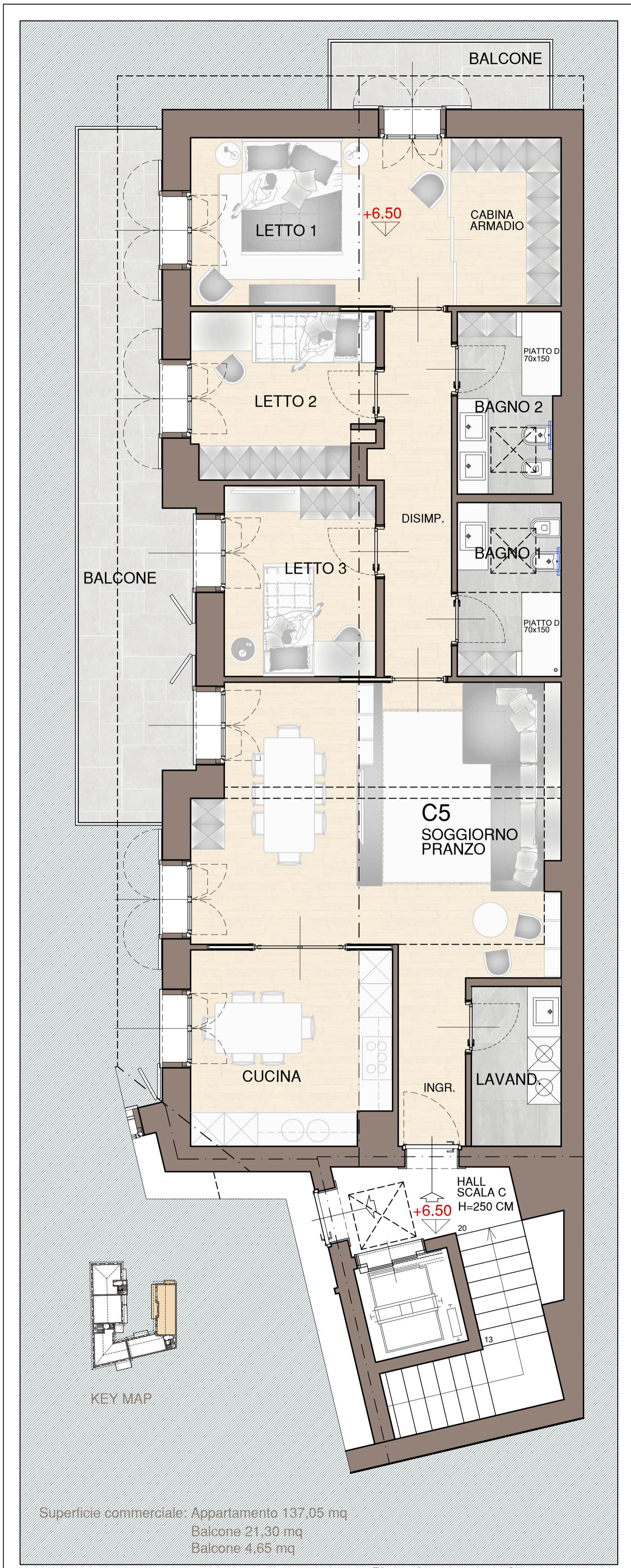
Pianta Appartamento C5 scala 1:50
